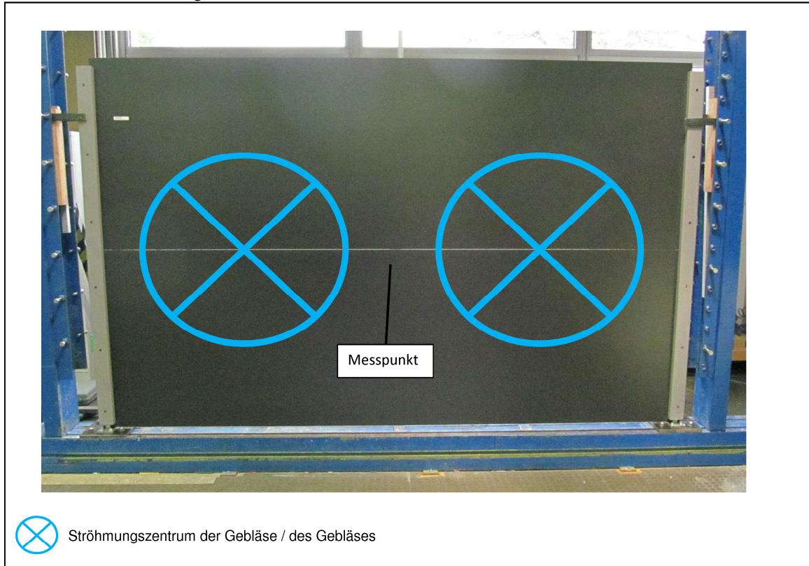
Darstellung: Gebläsepositionierung
