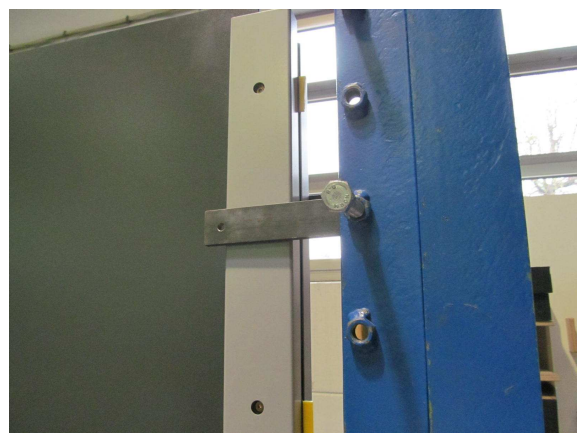
Bild 8 Seitliche Einspannung des Probekörpers als Abstützung zum Prüfstand
